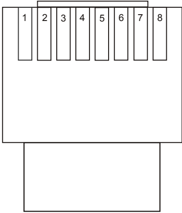
RJ 45 Draufsicht Kontakte sichtbar
